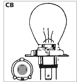
P43T (SA)
