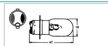
P15D-1
